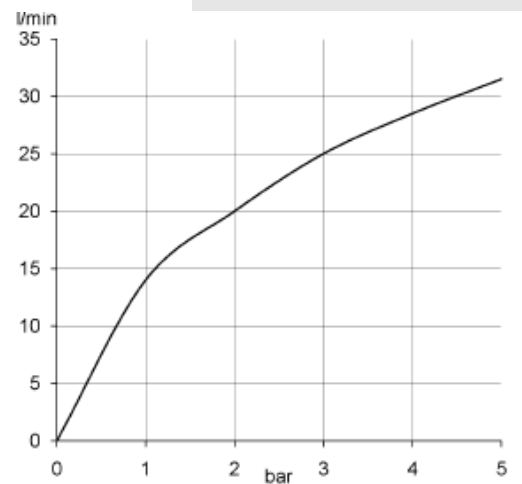
Durchflussdiagramm
