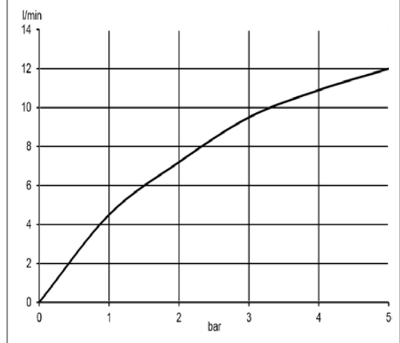
Durchflussdiagramm
