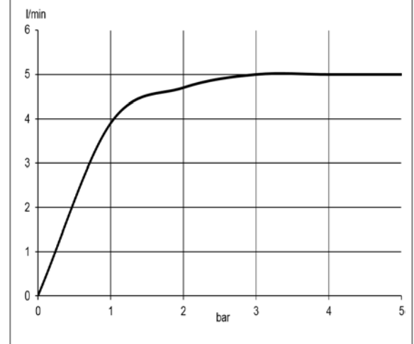
Durchflussdiagramm
